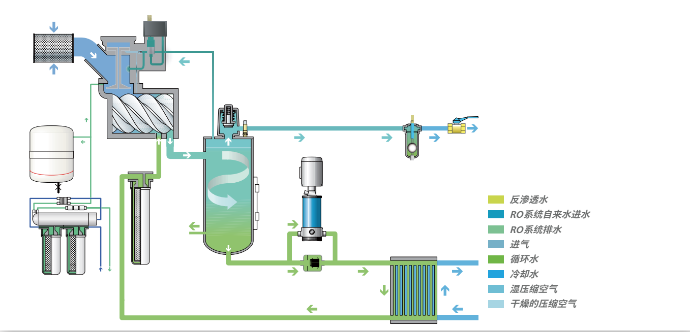
水冷式 AQ 流程图
