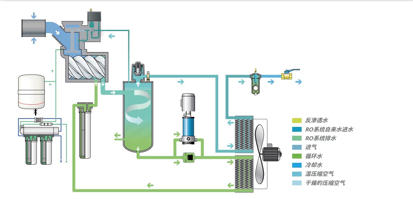
风冷式 AQ 流程图
